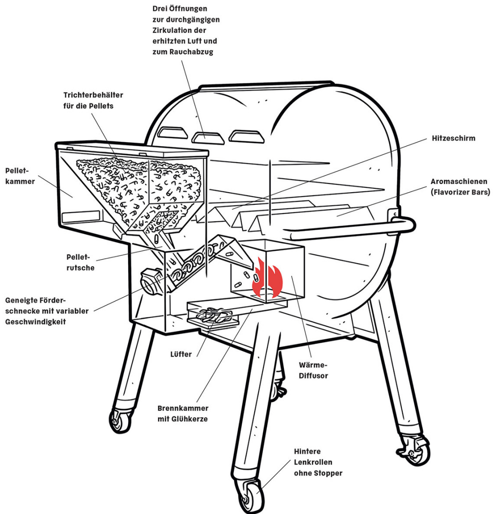
Rückansicht Pelletgrill
