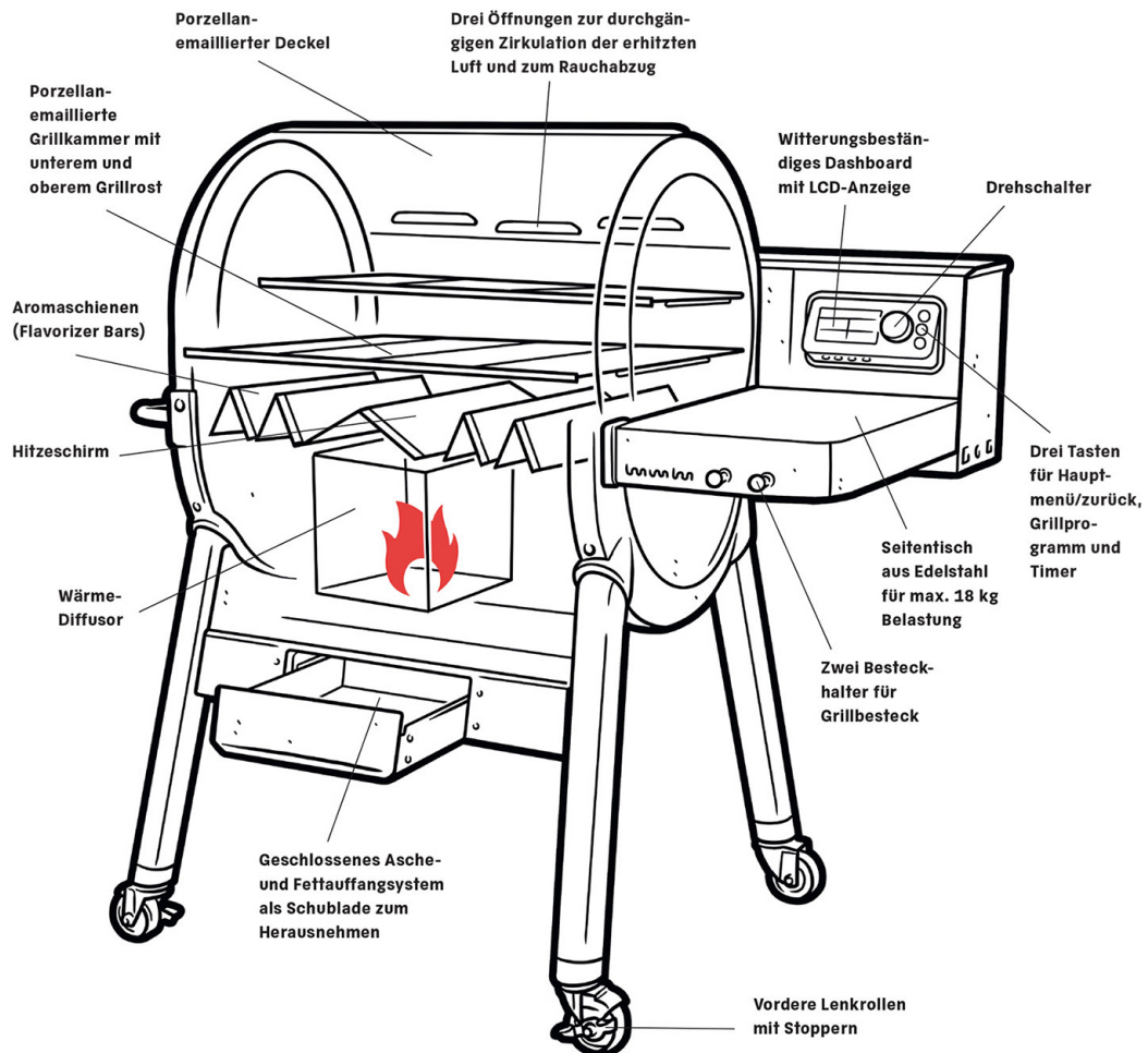
Vorderansicht Pelletgrill
